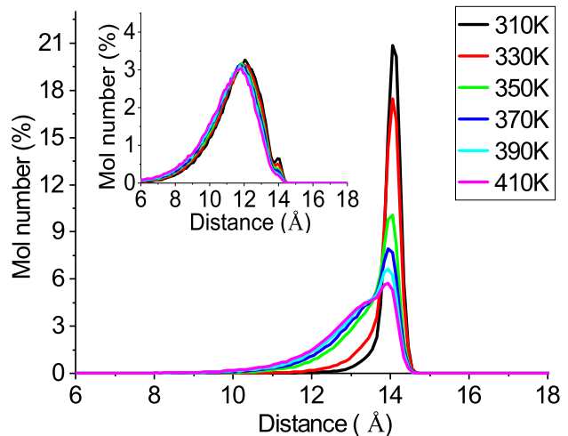
(d) PDF of end-to-end intramolecular distance of dodecane
