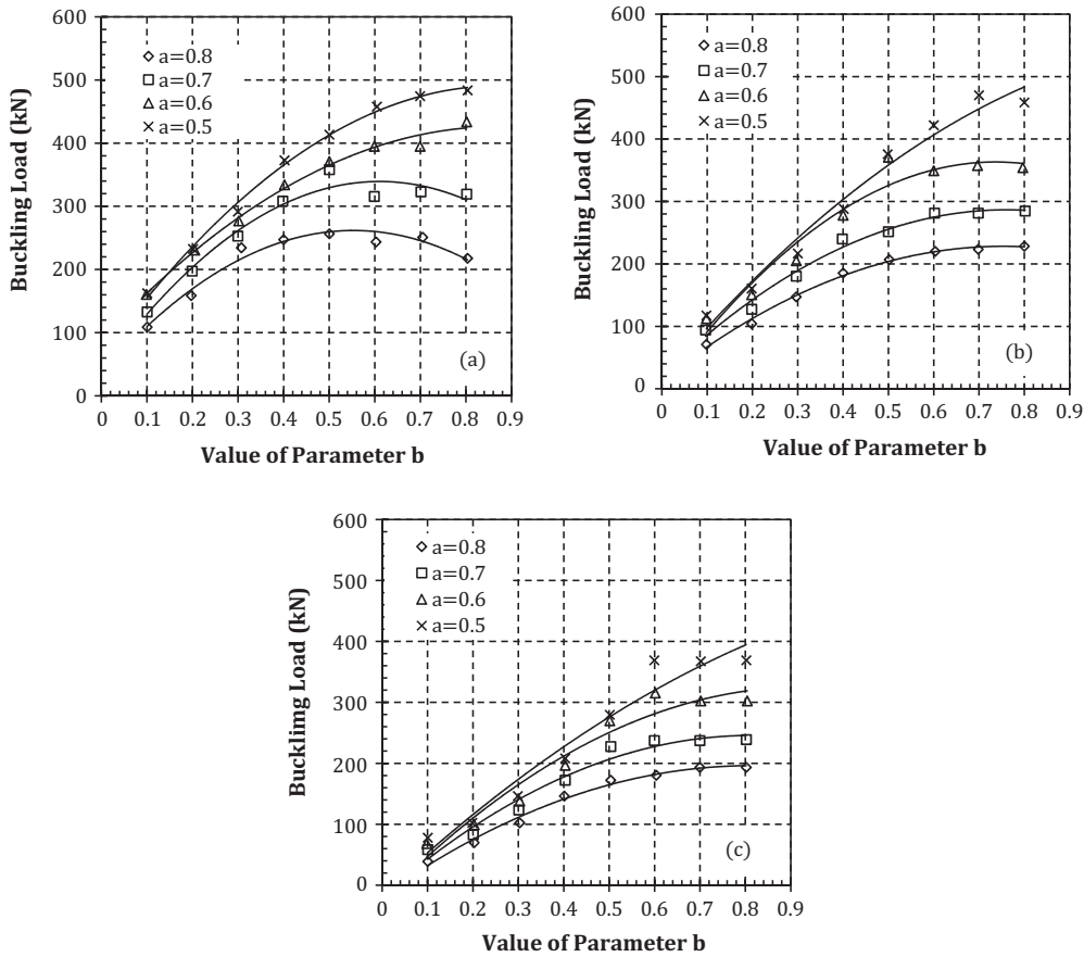
Fig. 19. Shear buckling capacities: (a) parameter c = 1.0 , (b) parameter c = 1.5 , (c) parameter c = 2.0 .
